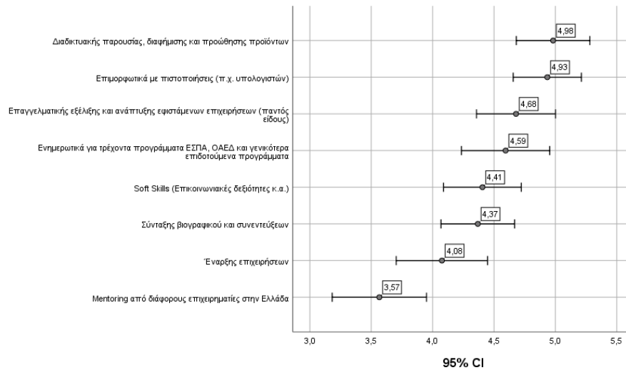
Εικόνα 7 95% διαστήματα εμπιστοσύνης για τον μέσο - Επαγγελματική απασχόληση - Σεμινάρια.
