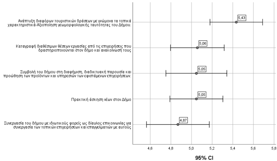
Εικόνα 5 95% διαστήματα εμπιστοσύνης για τον μέσο - Επαγγελματική απασχόληση – Συμβολή του δήμου Δομοκού.
