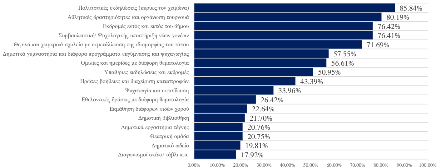
Εικόνα 12 Γραφική αναπαράσταση αξιολογήσεων ενδιαφέροντος – Ψυχαγωγία.
