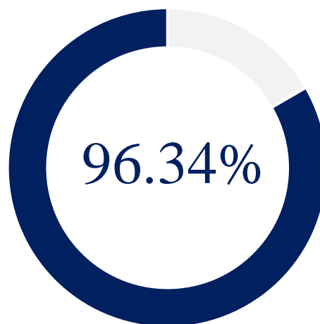
Εικόνα 1 Donut chart σχετικών συχνοτήτων επί τις % - Συναίνεση συμμετοχής στην έρευνα.
