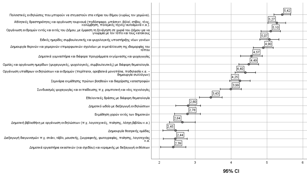
Εικόνα 11 95% διαστήματα εμπιστοσύνης για τον μέσο - Ψυχαγωγία.
