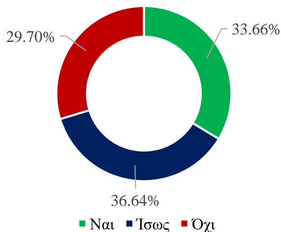
Εικόνα 4 Donut Chart σχετικών συχνοτήτων επί τις % - Εάν ΔΕΝ είστε ελεύθερος/η επαγγελματίας, θα σας ενδιέφερε μελλοντικά να κάνετε έναρξη επαγγελματικής δραστηριότητας;
