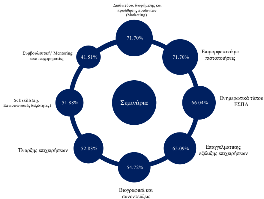
Εικόνα 8 Γραφική αναπαράσταση αξιολογήσεων ενδιαφέροντος - Επαγγελματική απασχόληση/ Σεμινάρια.
