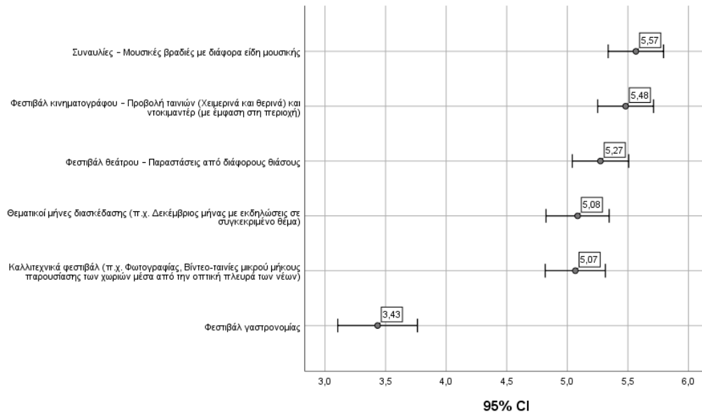
Εικόνα 13 95% διαστήματα εμπιστοσύνης για τον μέσο - Διασκέδαση.
