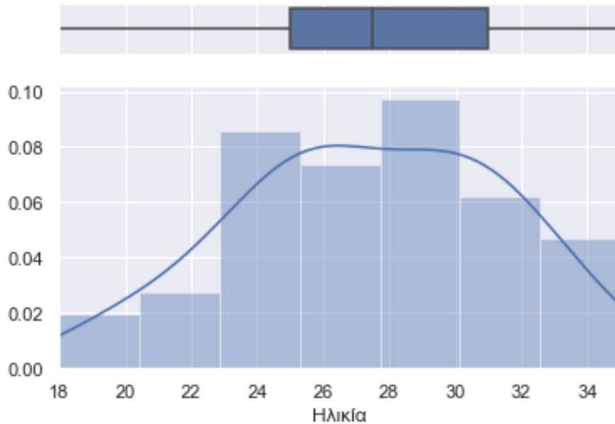
Εικόνα 2 Ιστόγραμμα κατανομής με εκτιμητή κατανομής πυρήνα KDE (Kernel Density Estimator) / Θηκόγραμμα κατανομής – Ηλικία.
