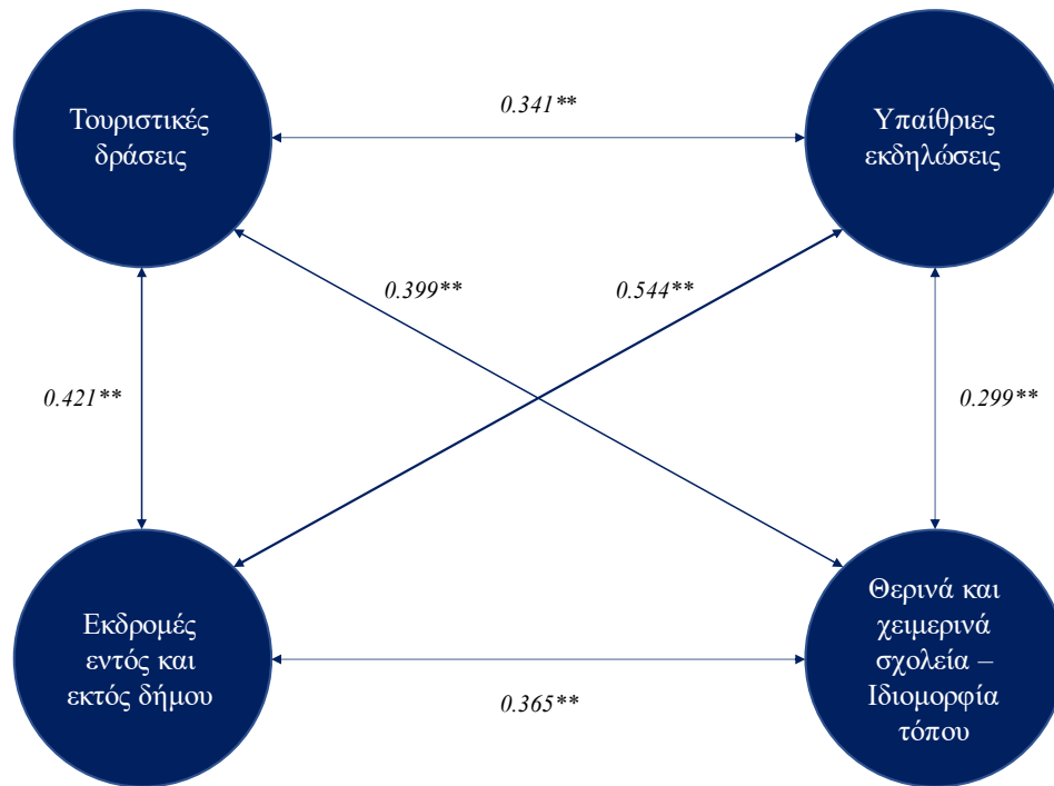
Εικόνα 15 Γραφική αναπαράσταση στατιστικά σημαντικών μη-παραμετρικών συσχετίσεων - Ανάπτυξη διάφορων τουριστικών δράσεων με γνώμονα τα τοπικά χαρακτηριστικά - Αξιοποίηση γεωμορφολογικής ταυτότητας του Δήμου / Οργάνωση υπαίθριων εκδηλώσεων και εκδρομών (περίπατοι, ορειβατικά μονοπάτια, ποδηλασία κ.α. – δημιουργία συλλόγων) / Οργάνωση εκδρομών εντός και εκτός του Δήμου, με έμφαση τη ξενάγηση σε χωριά του Δήμου για να γνωριμία με τον τόπο και τους κατοίκους / Δημιουργία θερινών και χειμερινών επιμορφωτικών σχολείων με εκμετάλλευση της ιδιομορφίας του τόπου.
