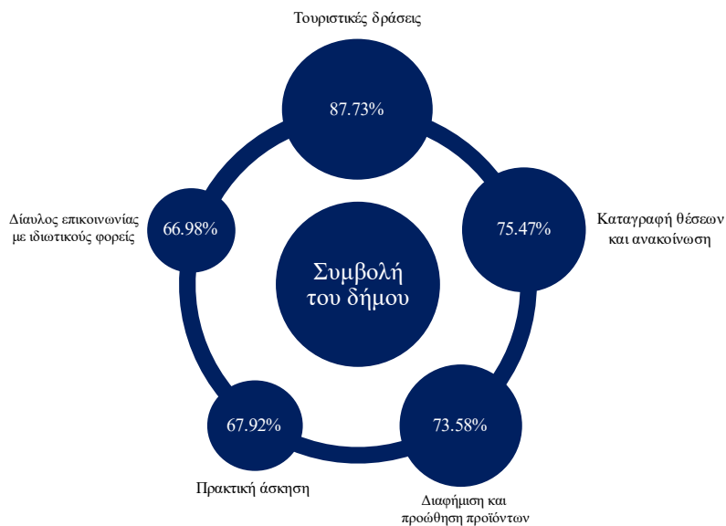
Εικόνα 6 Γραφική αναπαράσταση αξιολογήσεων σημαντικότητας - Επαγγελματική απασχόληση/ Συμβολή του δήμου.
