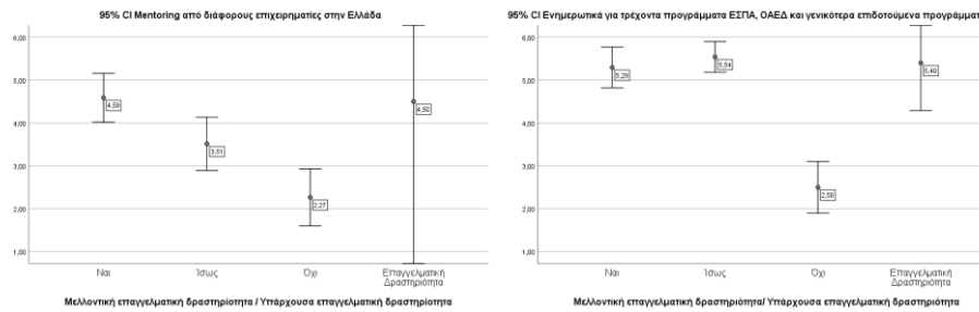
Εικόνα 10 95% διαστήματα εμπιστοσύνης για τον μέσο - Επαγγελματική απασχόληση/ Σεμινάρια -Μελλοντική επαγγελματική δραστηριότητα/ Υπάρχουσα επαγγελματική δραστηριότητα.
