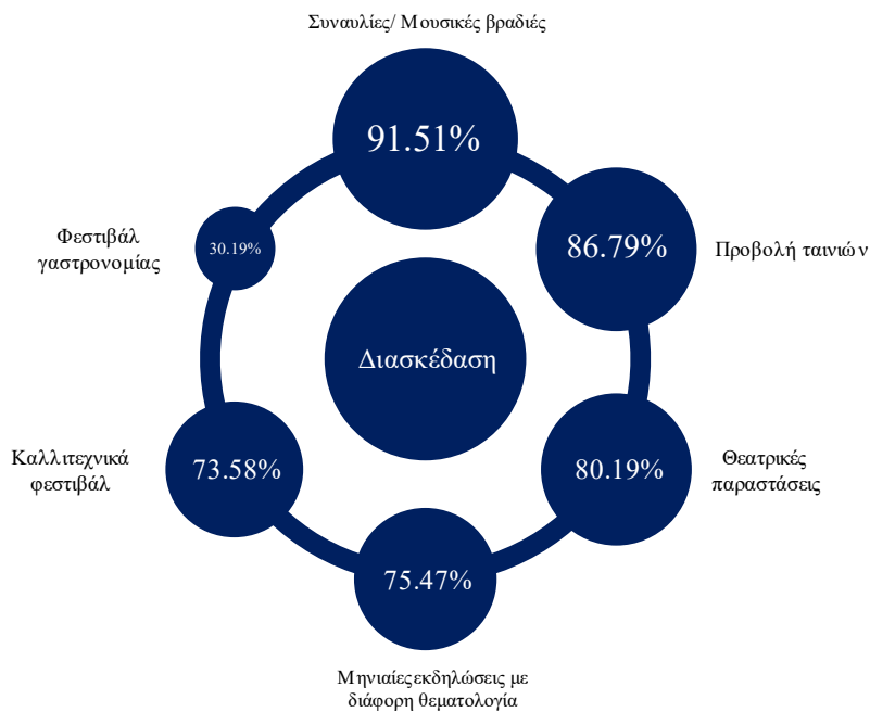
Εικόνα 14 Γραφική αναπαράσταση αξιολογήσεων ενδιαφέροντος – Διασκέδαση.
