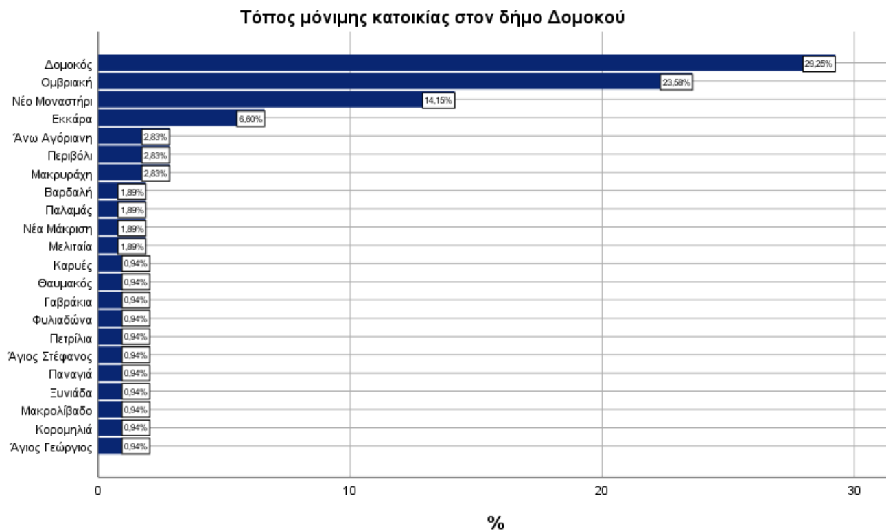
Εικόνα 3 Συγκριτικό ραβδόγραμμα σχετικών συχνοτήτων επί τις % - Τόπος μόνιμης κατοικίας.
